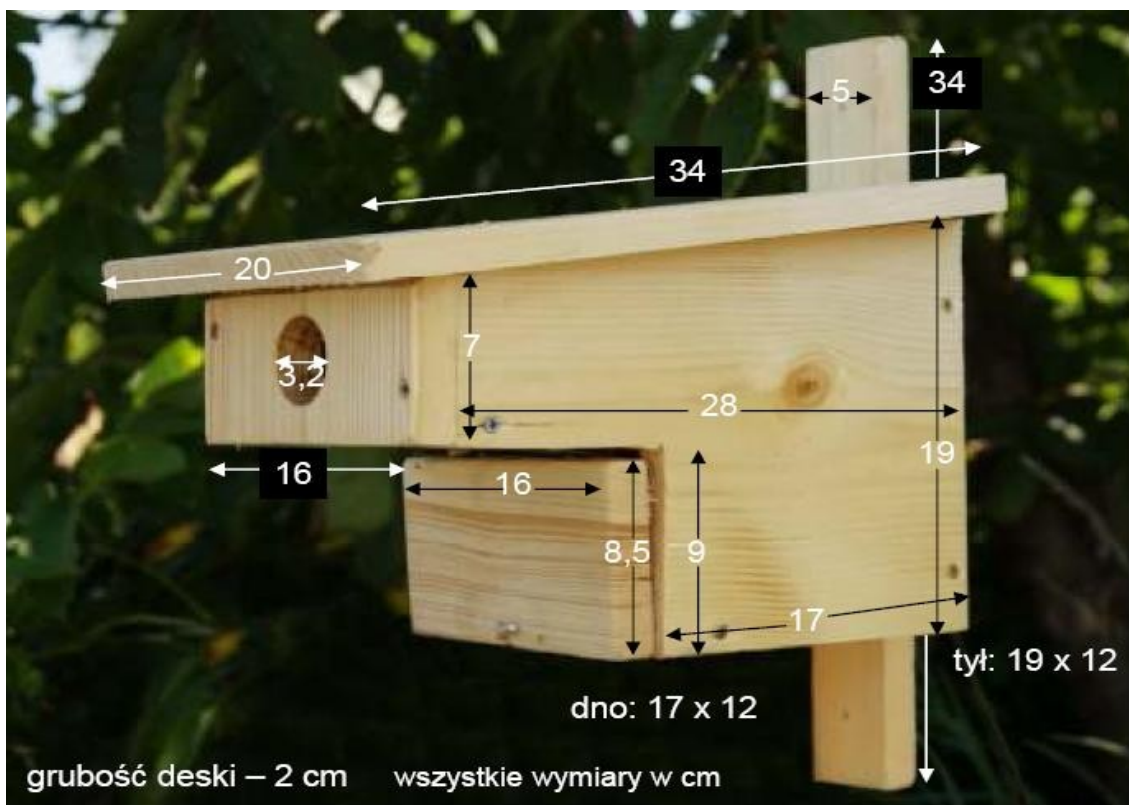
Ryc. 1. Schemat budki lęgowej dla wróbli.
